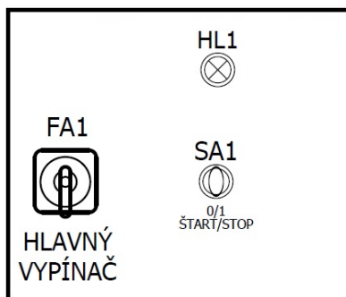
Príklad umiestnenia prvkov na rozvádzači
